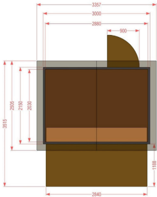
Datenblatt Rustikale Markthütte „3m-Hütte“ 3,00m x 2,15m
